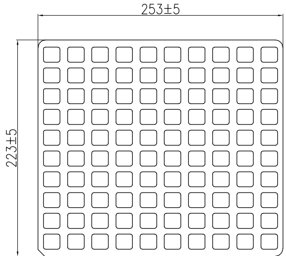
吸塑盒底盘
